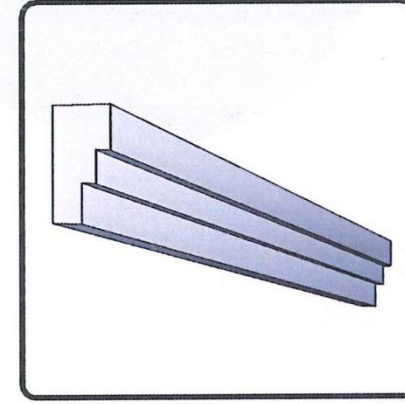
LRC - COR 1032 50(D) x 100(H) x 1000(L)
