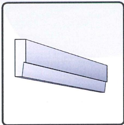
LRC - COR 1029 30(D) x 130(H) x 1000(L)
